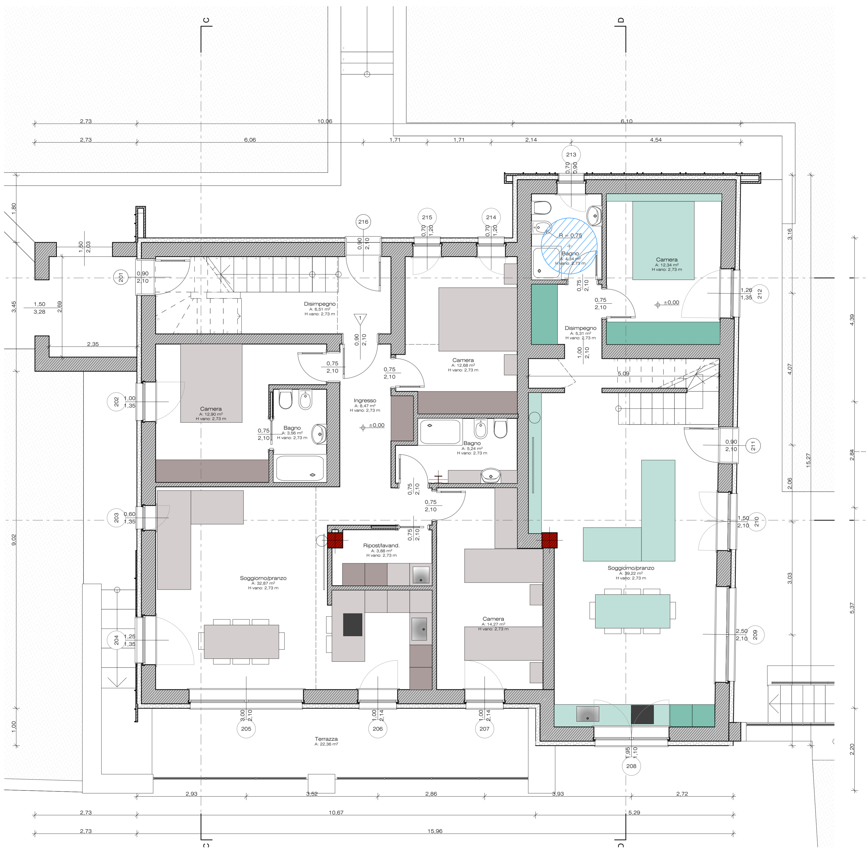
PIANTA PIANO TERRA
