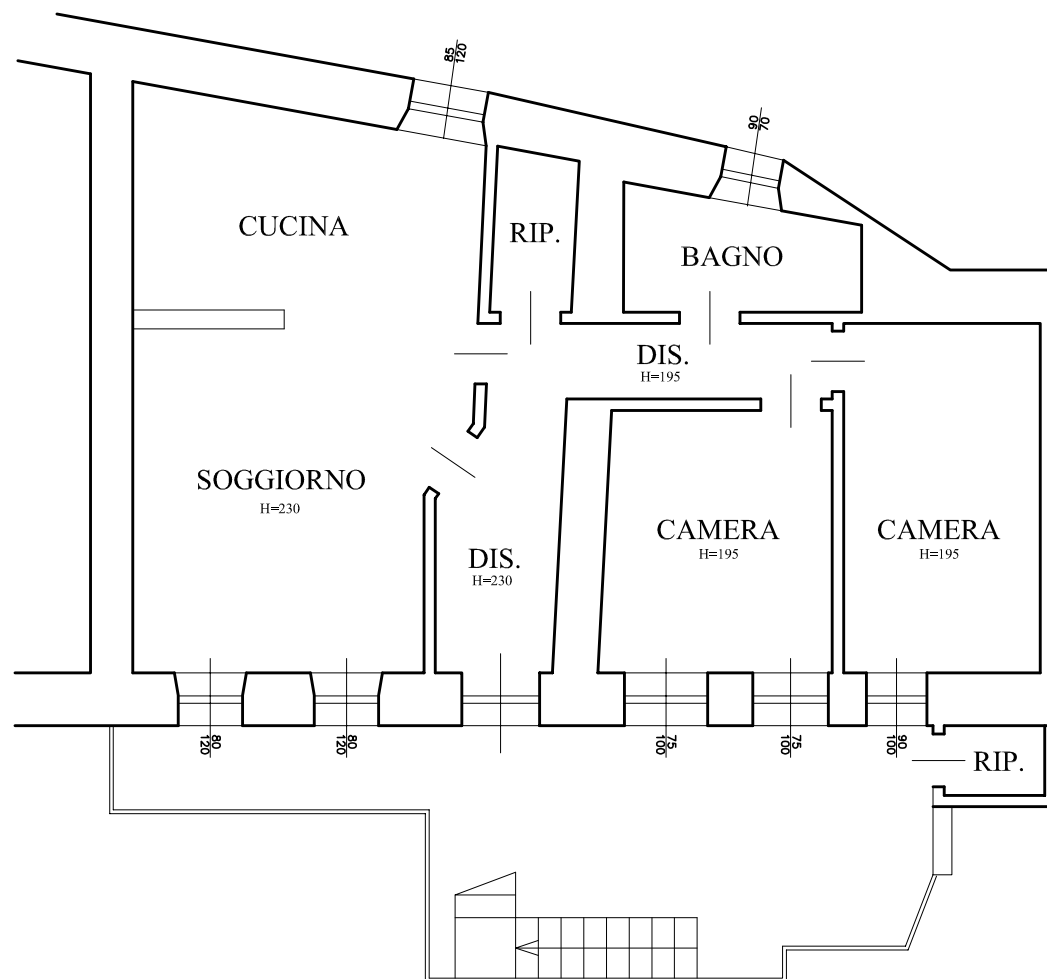
RILIEVO PIANTA PIANO TERRENO
