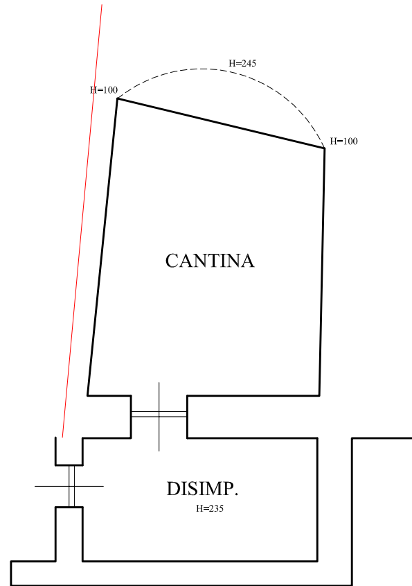
RILIEVO PIANTA PIANO INTERRATO
