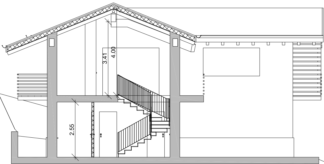
SEZIONE B - B Scala 1:100
