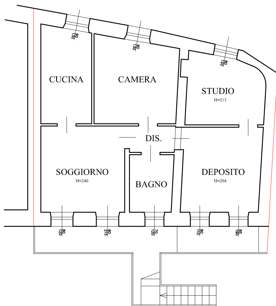
RILIEVO PIANTA PIANO PRIMO
