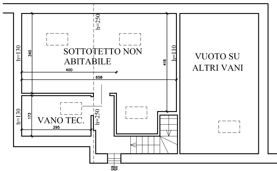
PIANTA DI RILIEVO PIANO SOTTOTETTO
