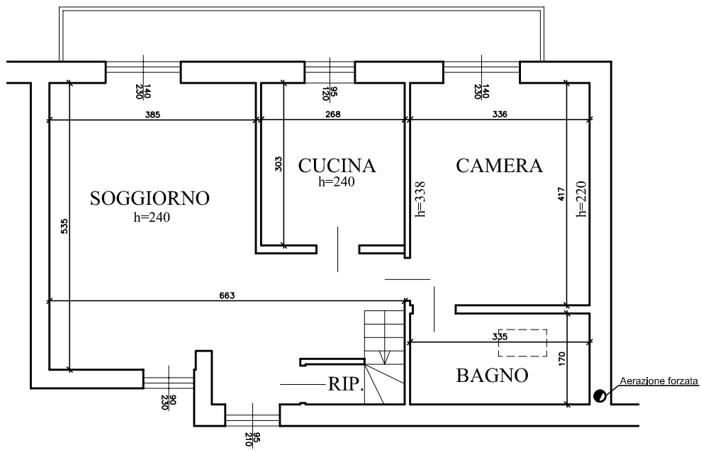
PIANTA DI RILIEVO PIANO PRIMO
