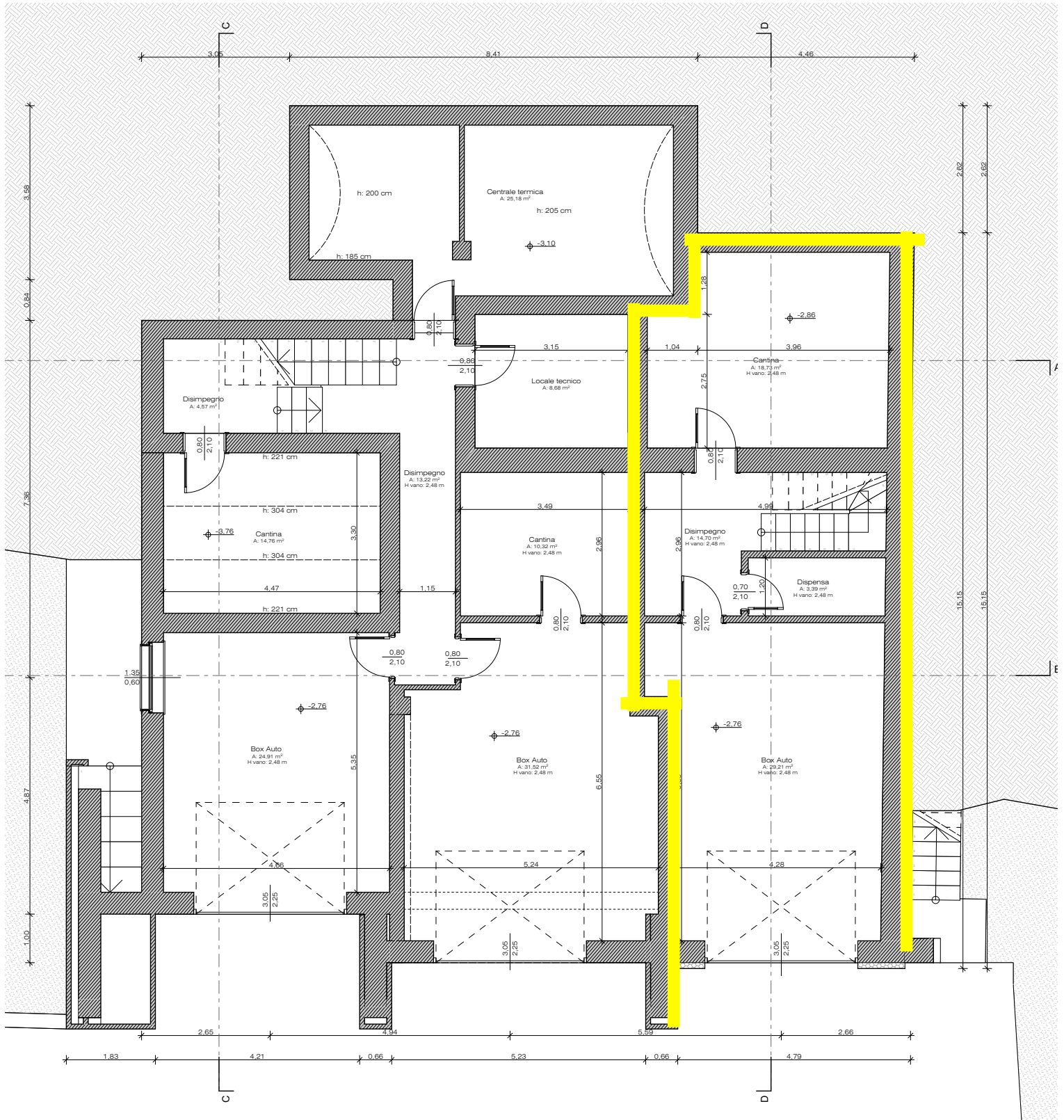
PIANTA PIANO SEMINTERRATO
